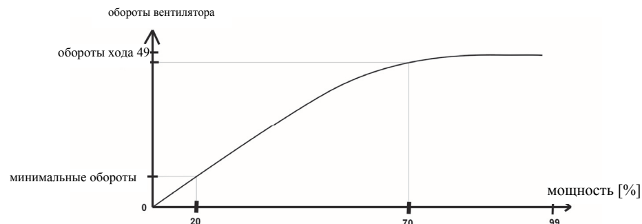
Оптимальный диапазон производительности вентилятора
